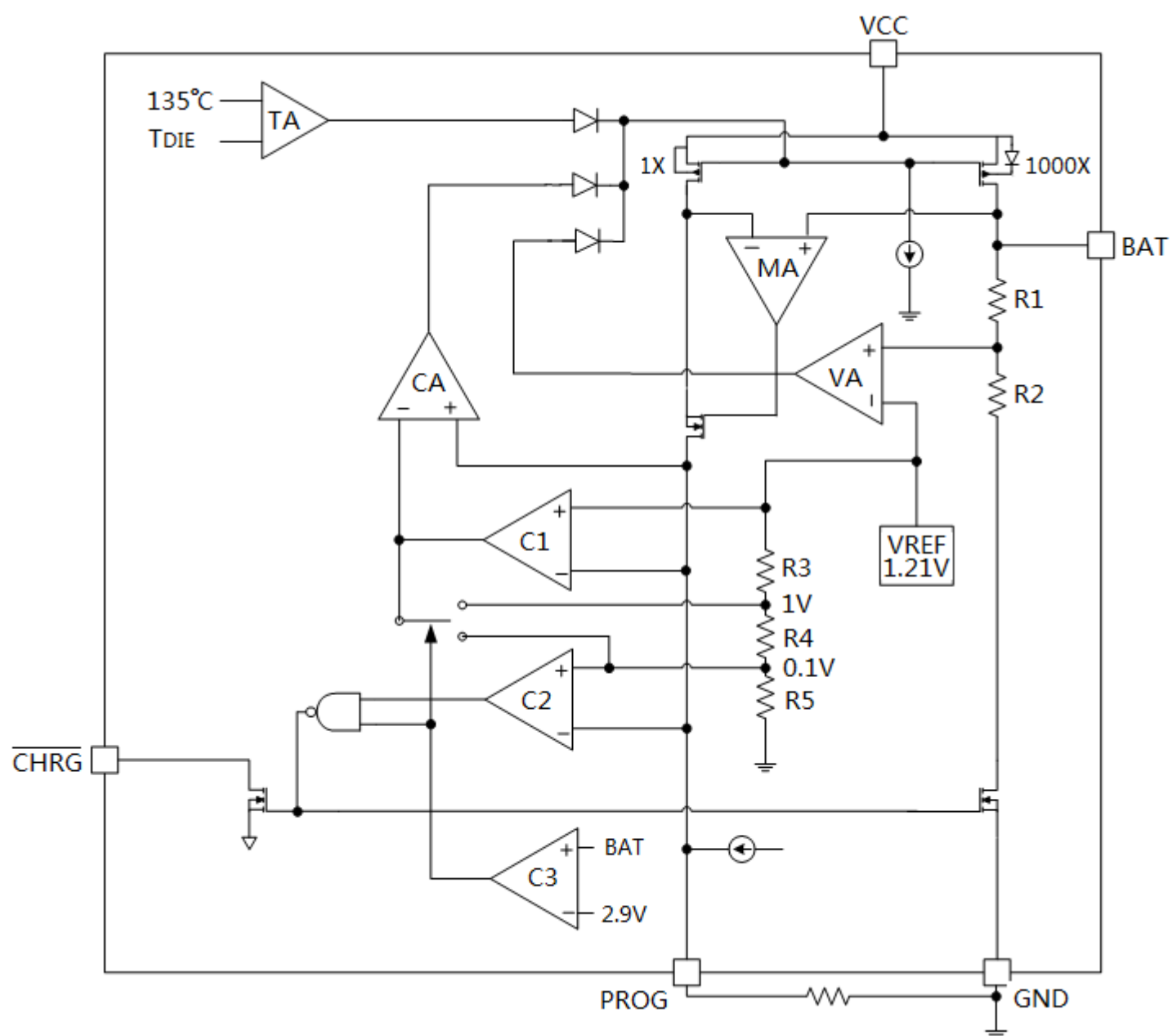
结构框图
